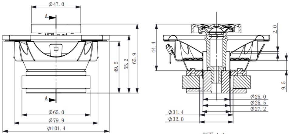
剖面 A-A 比例 1 : 1.3
